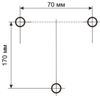
Рисунок 1. Крепление громкоговорителя
